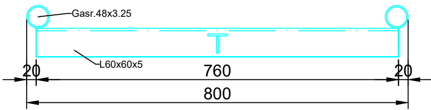
Schnitt Abschlusswinkel
