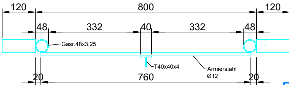
Schnitt Armierstahl
